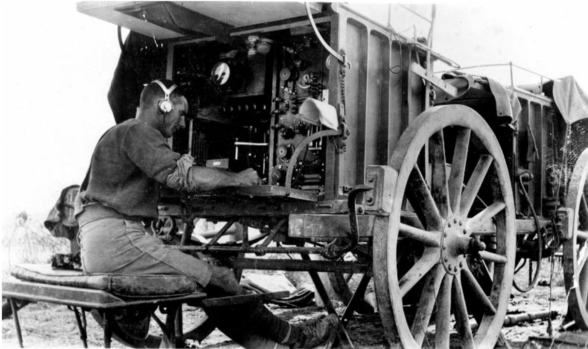
Fig. 103 - Operatore di una stazione radio trasportabile della Marconi installata su un carro durante la prima guerra mondiale.
