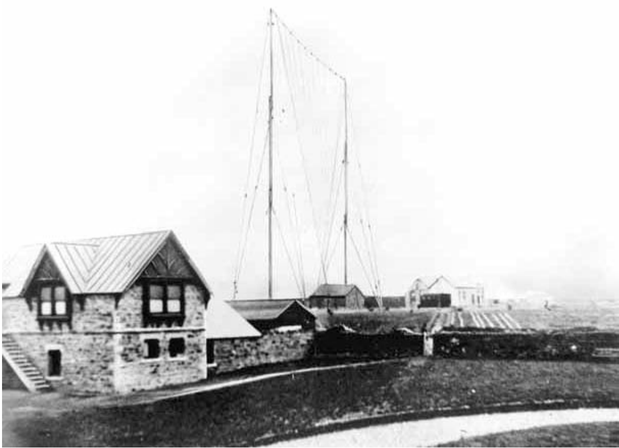
Fig. 46 - L'antenna di Poldhu dopo la ricostruzione, che ha permesso il primo collegamento radio transatlantico. Essa è composta da due piloni alti 45 m che sostengono 55 fili convergenti in basso.
