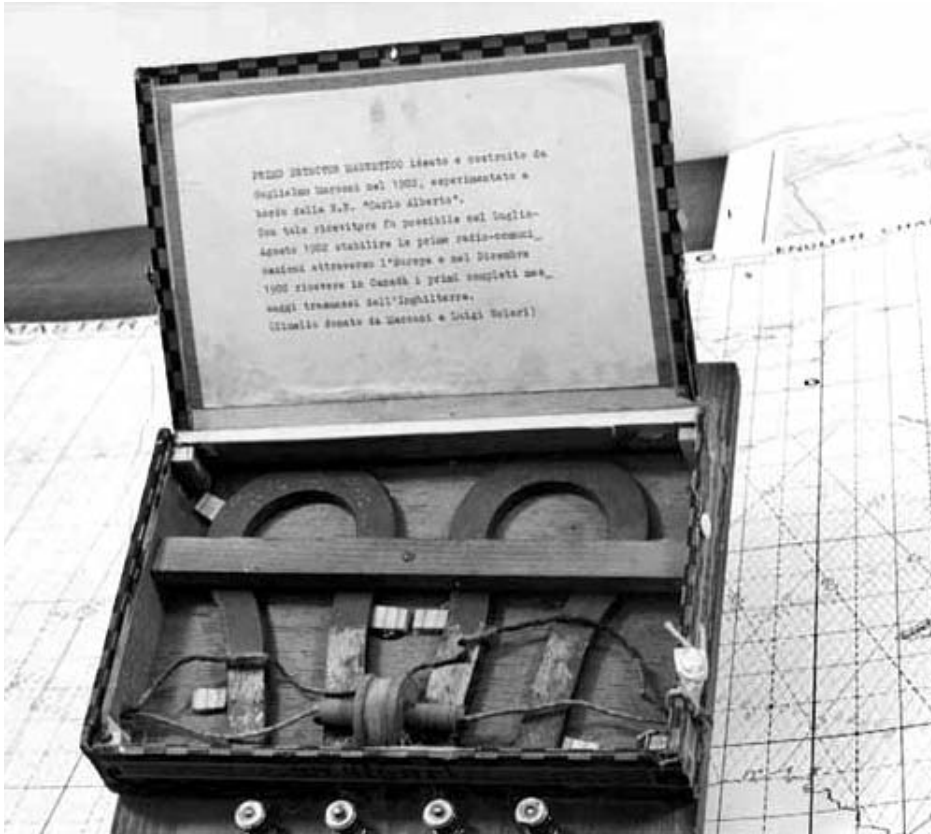
Fig. 57 - Primo detector magnetico costruito personalmente da Marconi assemblando i componenti in una scatola di sigari. Il filo che passa attraverso la bobina viene azionato manualmente.
