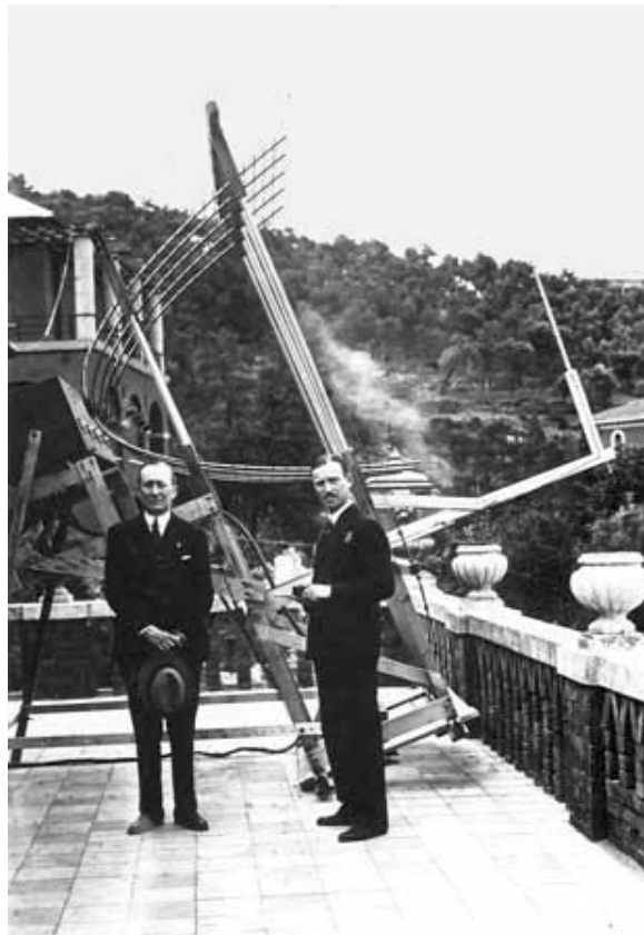
Fig. 134 - Marconi e il suo assistente Mathieu nella postazione dell'antenna a microonde installata nella Città del Vaticano.
